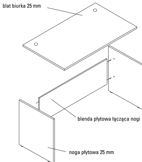
KONSTRUKCJA STELAŻA - OPCJA "2"
