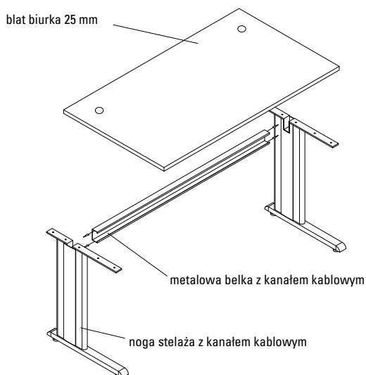
KONSTRUKCJA STELAŻA - OPCJA "1"
